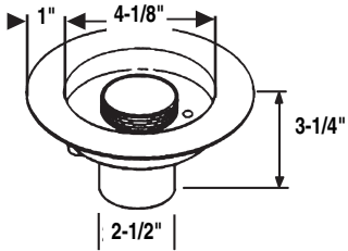
119-1630-SR
